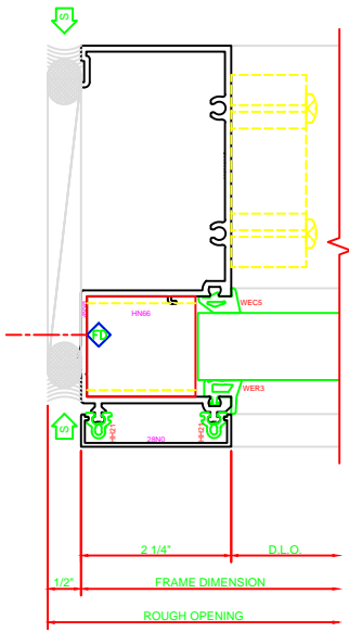
400 JAMB SERIES: 600R
